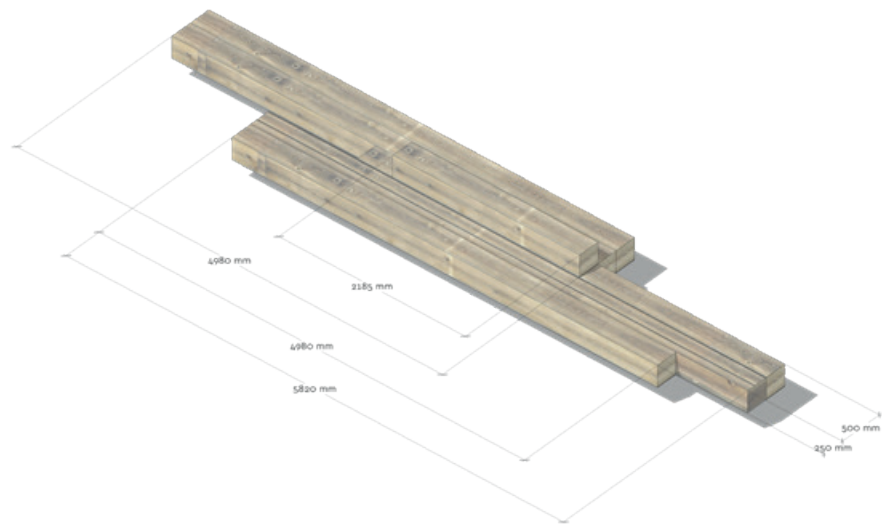
Парковая скамья. Тип-4 из цельного бруса с дополнительной секцией.
