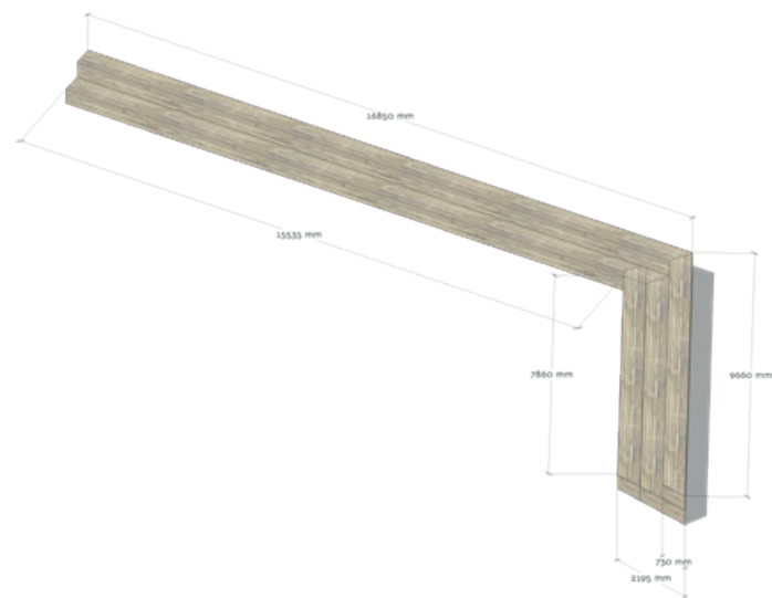
Парковая скамья. Тип-5 из цельного бруса.
