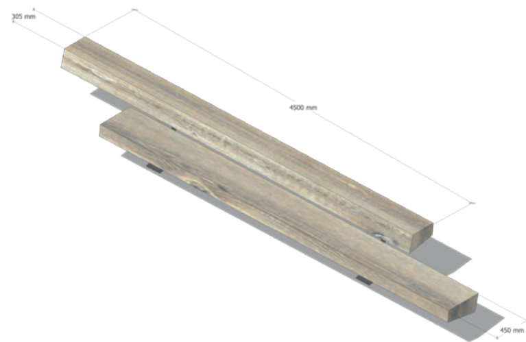
Парковая скамья. Тип-2 из цельного бруса
