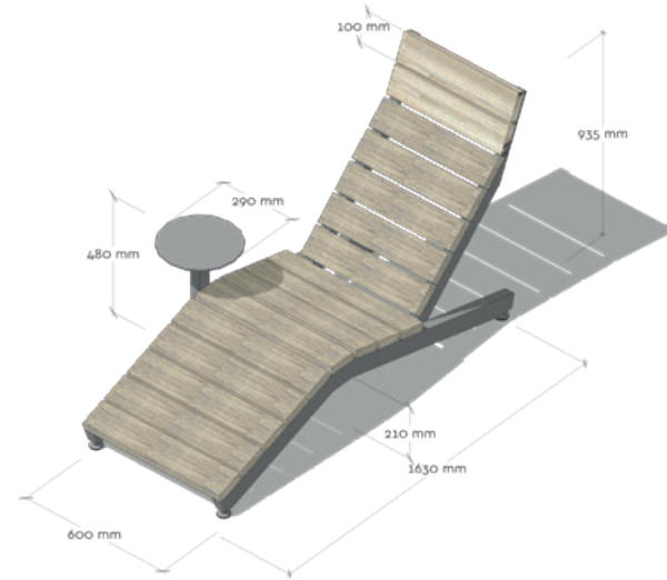
Шезлонг. Тип-1. С интегрированным столиком
